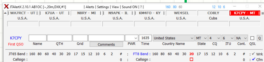
JTAAlert
